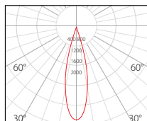
FARETTO SPOT 5W - 24°
