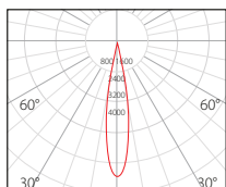
FARETTO SPOT 7W - 24°
