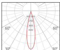
FARETTO SPOT 12W - 24°
