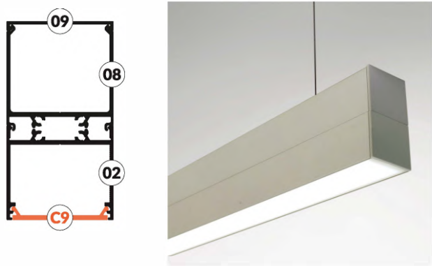
variant 27 - pendant 09-08-02-C9
