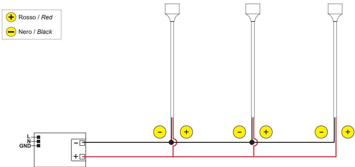
Schema di connessione in parallelo per versione 24V - Connection diagram for 24V version
