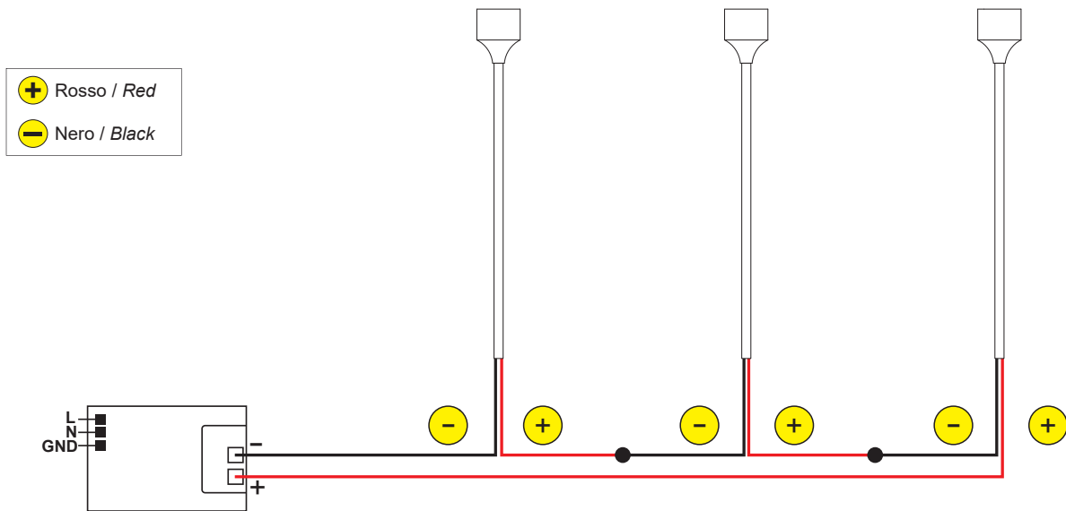
Schema di connessione in serie per versione 700mA - Connection diagram for 700mA version
