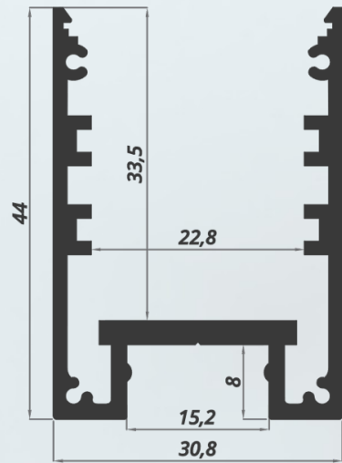
Profilo dissipatore led in alluminio (Consigliato l'utilizzo con strip LED fino a 30 W/m )
