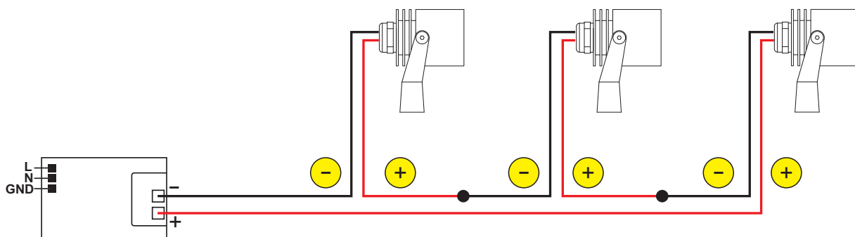
Schema di connessione in serie per versione 500mA - Connection diagram for 500mA version
