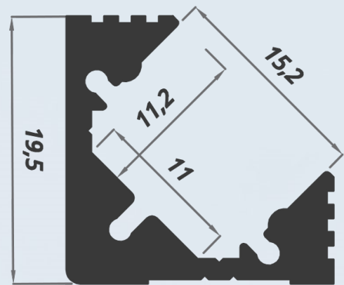
Profilo dissipatore led in alluminio da parete e angolo
