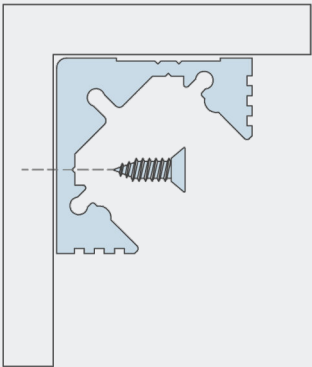
Vite su profilo
