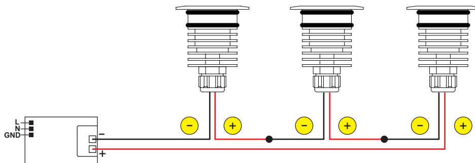
Schema di connessione in serie per versione 350 / 500mA Connection diagram for 350 / 500mA version
